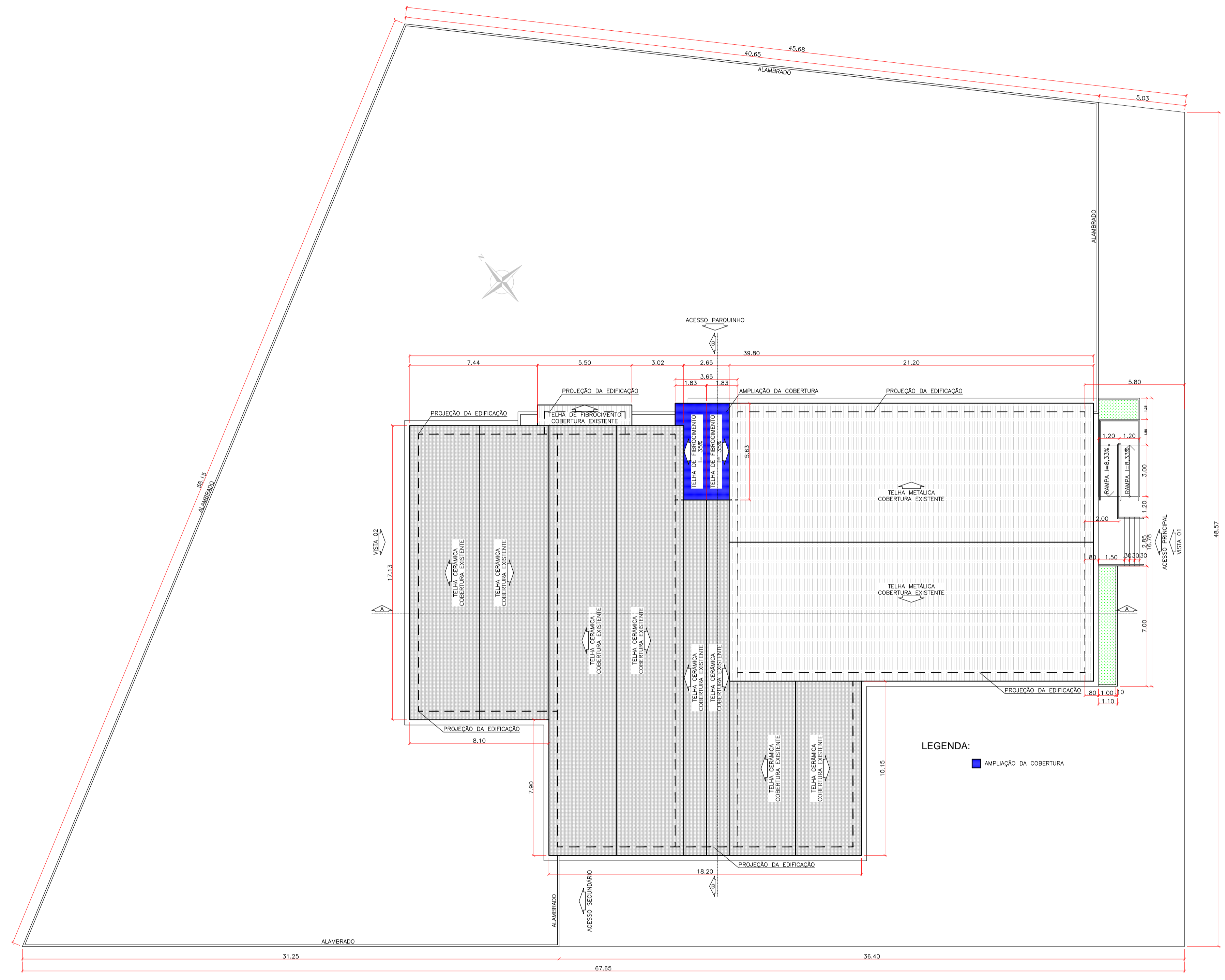
PLANTA BAIXA DE IMPLANTAÇÃO E AMPLIAÇÃO DA COBERTURA esc 1:150
