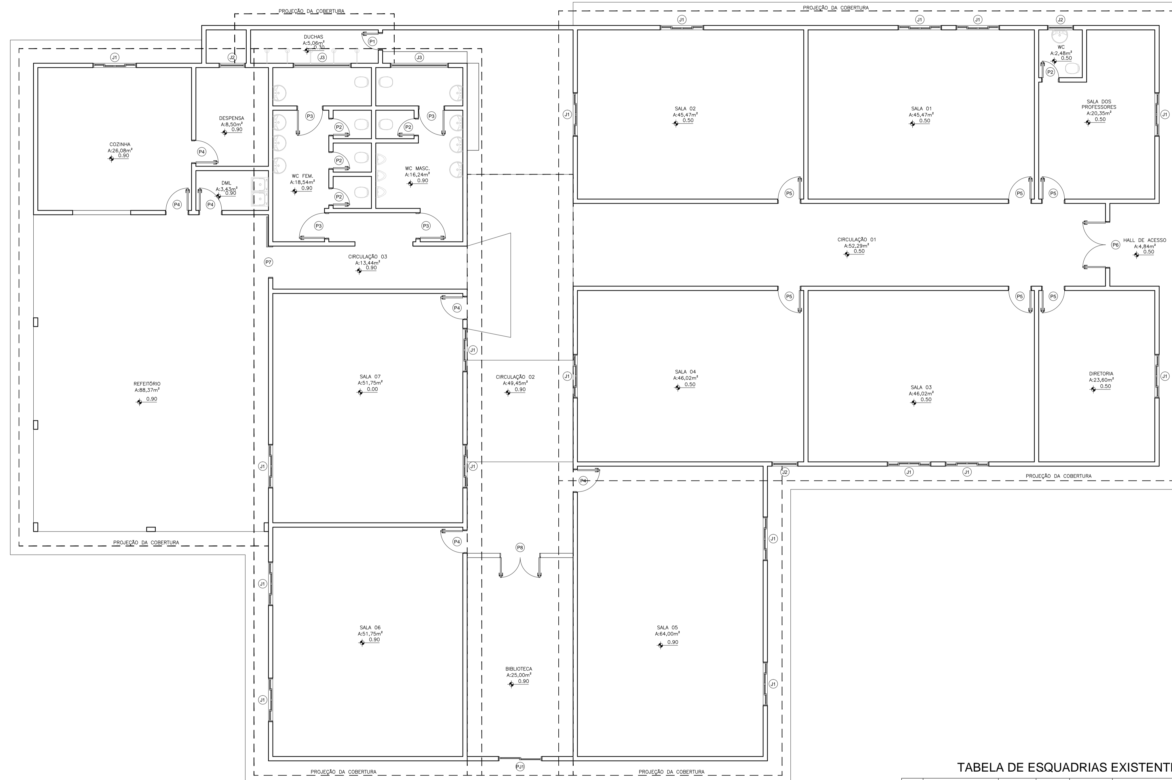
PLANTA BAIXA EXISTENTE esc 1:75
